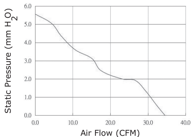
CFM-7025B-140-394
