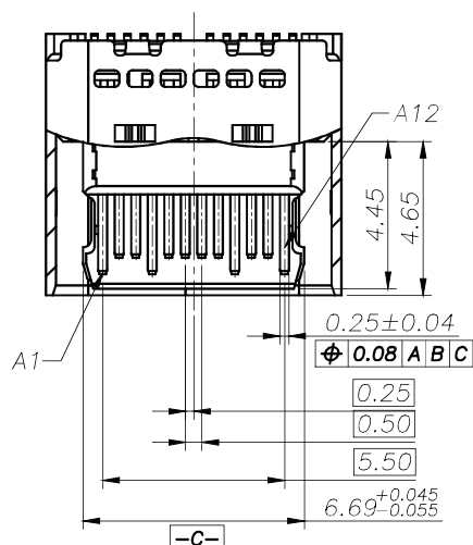
SECTION:D-D SCALE 1:1
