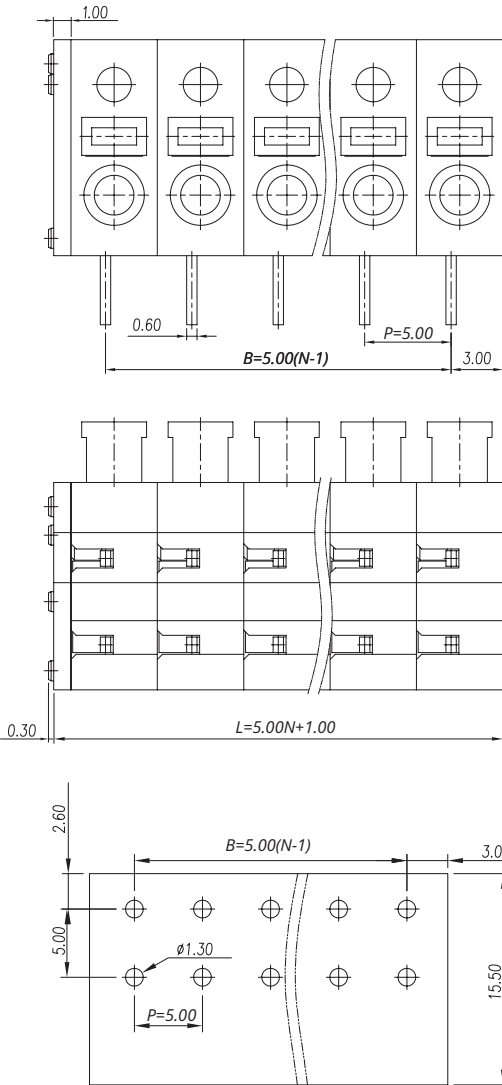
P.C.B. LAYOUT
