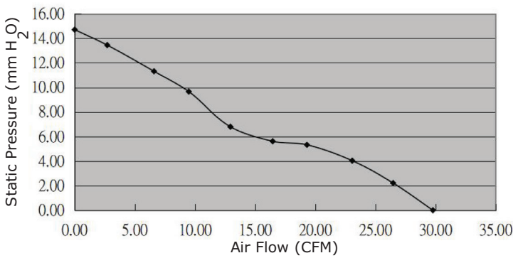
CFM-6025BG68-170-434
