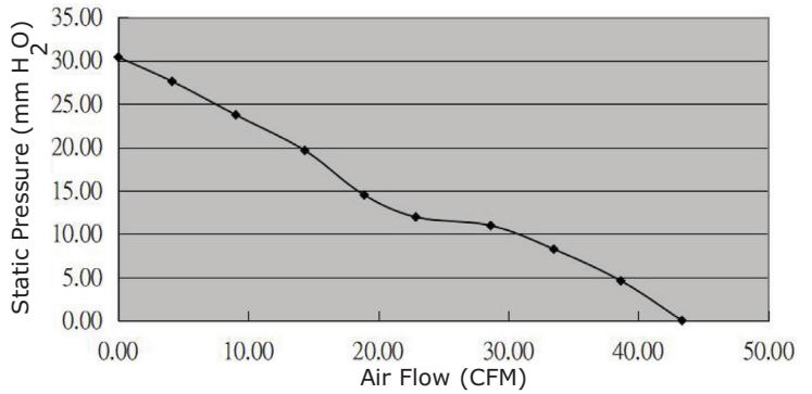
CFM-6025BG68-1100-535
