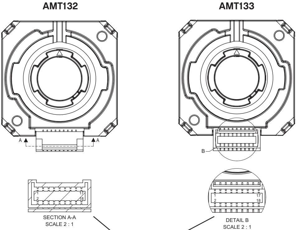
Mating Connector: JST ZPDR-18V-S
