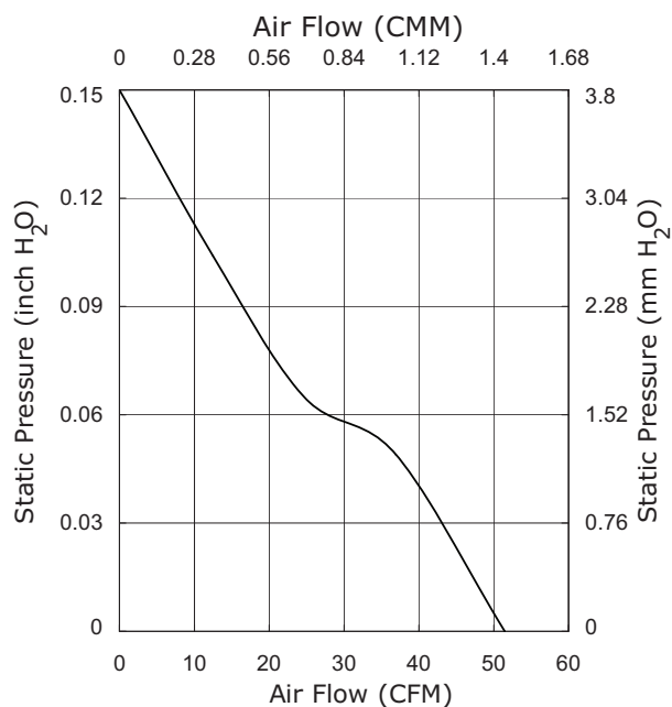
CFM-9225V-230-340
