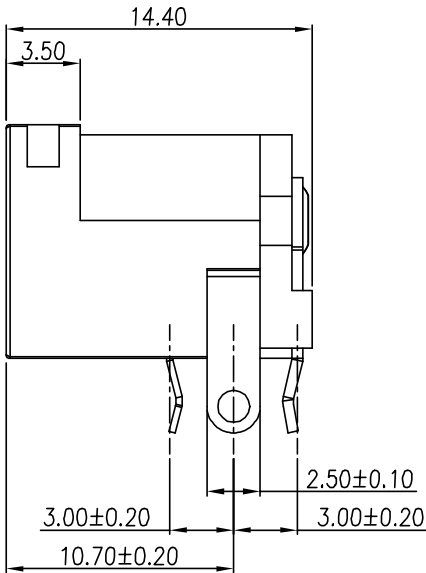
SEC: A-A
