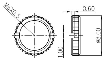
Nut
