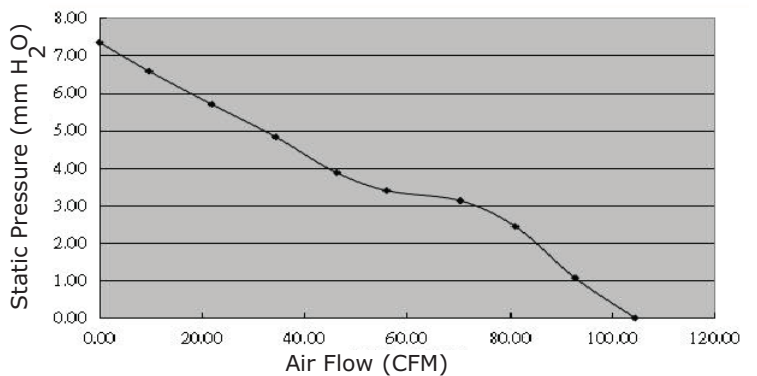
CFM-A225BG-430-459
